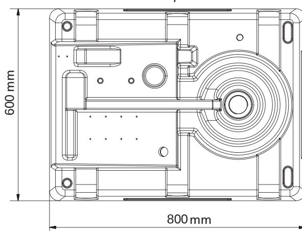
Vista dall'alto - Top view - Vue de dessus
