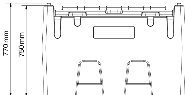
Vista laterale - Lateral view - Vue latérale
