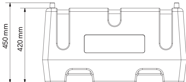
Vista laterale - Lateral view - Vue latérale
