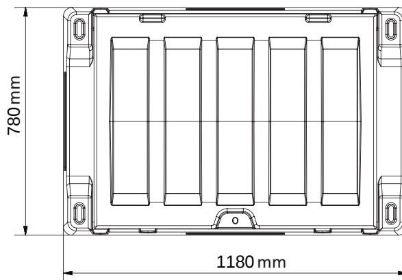
Vista dall'alto - Top view - Vue de dessus
